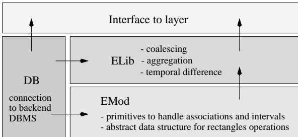
Fig. 7.21. The external modules
